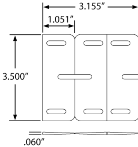
HS 350 BP 3½" QUICK ALIGN HINGE SHIM
